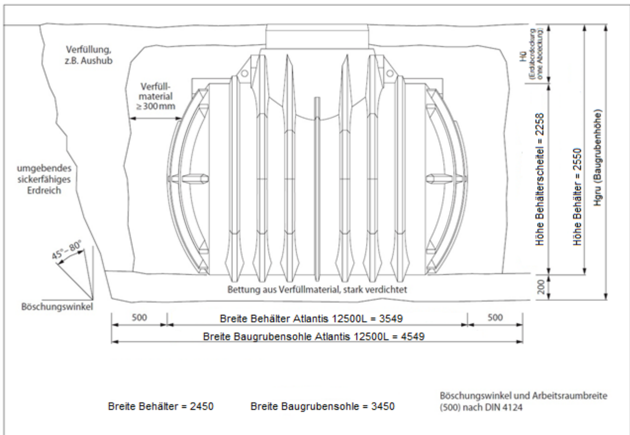
Abbildung 2: Einbaugrößen
